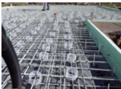
Abb. 2: Glasfasergitter vor dem Betonieren
